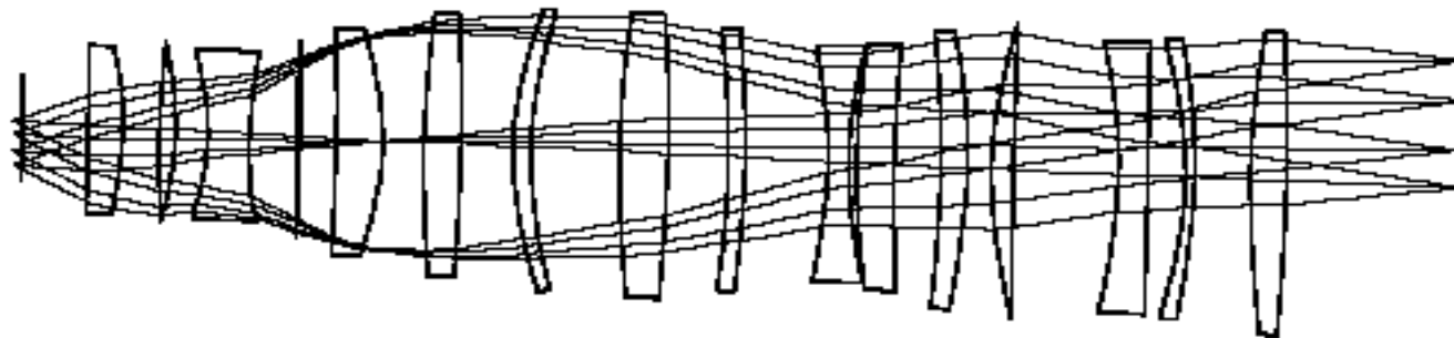
15枚組投影レンズ
